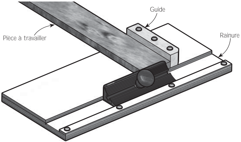
Figure 2 : Exemple d'une planche à recaler maison
