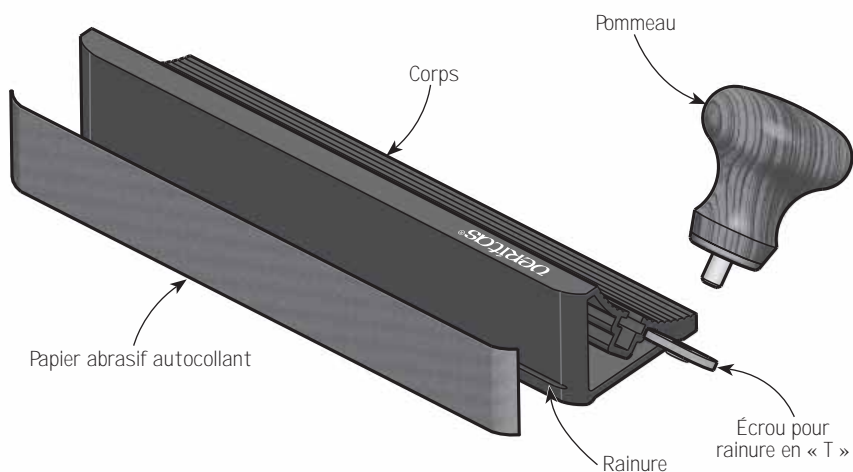
Figure 1 : Cale de ponçage pour planche à recaler Veritas
